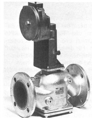
Neuheit an der Welt-Gasausstellung: Gasventil mit angebautem Gas/Luft-Verhältnisregler (Foto: Landis & Gyr).
