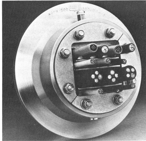
Neuheit an der Welt-Gasausstellung: Hochdruckdichtung für Bohrseln (Foto: AB Lyckeaborgs Bruk, Karlskrona).
