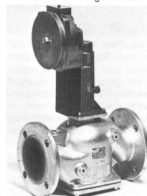
Neuheit an der Welt-Gasausstellung: Gasventil mit angebautem Gas/Luft-Verhältnisregler (Foto: Landis & Gyr).
