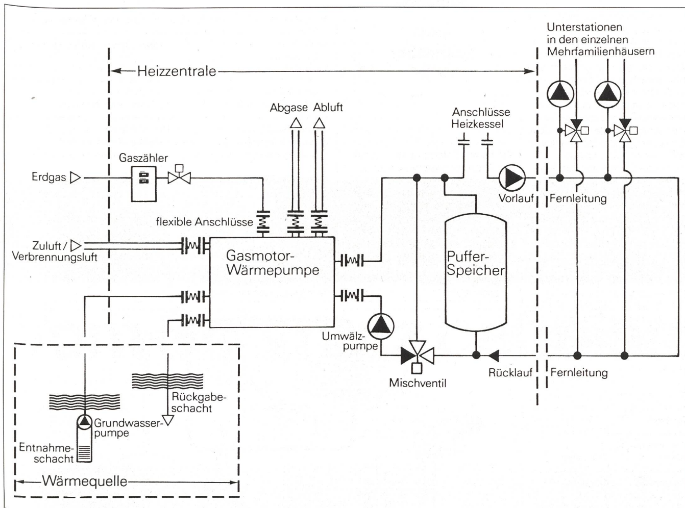
Abb. 2. Prinzipschema Gasmotorwärmepumpe mit Fernwärmeversorgung.
