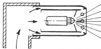
Warmluft-Spezialmischkopf.
