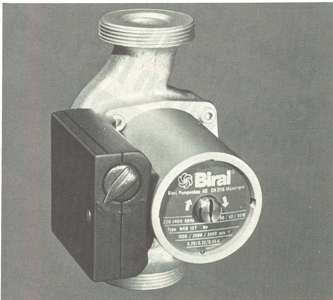
NRB 12T: Dreitourige Umwälzpumpe mit besonders grossem Anzugsmoment.
