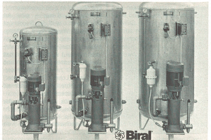
Neu: Druckwasserautomat DWA-K – wenn das Wasser nicht durch natürlichen Druck zufliesst, wenn das Wasser zuwenig Druck aufweist, wenn keine Wasserversorgung vorhanden ist.
