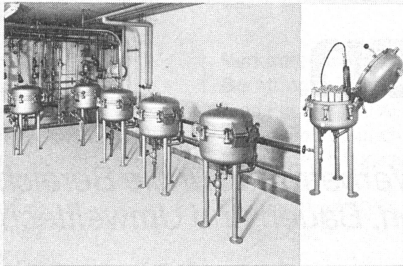
Ausschnitt aus einer Gruppe von 11 Entkeimungfiltern MF 31, Mineralquelle Eglisau, Leistung: 1000 l/min.
