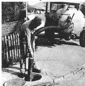
Schächte absaugen
