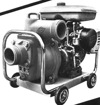
«Multus»-UV, Wasserversorgung Buchs SG, Leistung: 4000 l/min.
