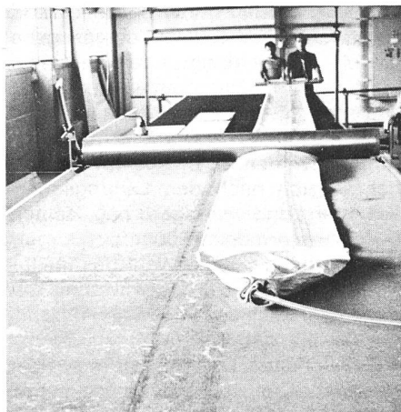
Abb. 3. Polyestergetränkter Filzschlauch im Endschacht vor dem Aushärten.
