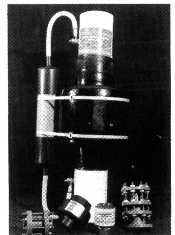
Ziefle-Monobloc-Isolierstück mit aufmontiertem Überspannungsableiter. Auswahl von Ziefle-Rohrleitungsbauteilen.
