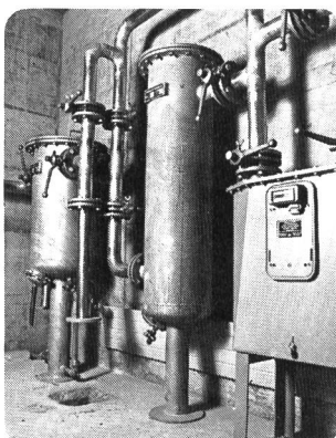
Trockengasometer und Gasreinigung (ARA, Wartau/SG)
