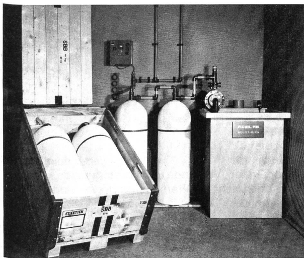
Mesil-Kompakt-Kreislaufanlage mit Reserve-Spiel Ionenaustauscheranlage MKK 75
