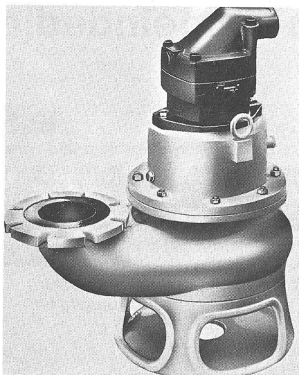
▲ Turo-Unterwasserpumpe mit hydraulischem Antrieb
