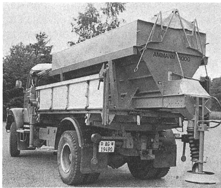
Gross-Streuer Ammann 6000 zum Aufsetzen auf Lastwagenbrücken, Behälterinhalt 6 m 3
