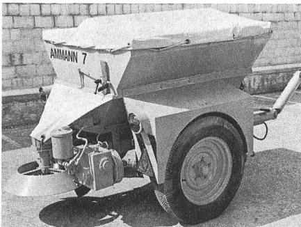
Anhängerstreuer Ammann 7, Behälterinhalt 0,75 m 3
