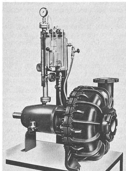
▲ Verschleissfeste Turo-Pumpe Bauform HN
