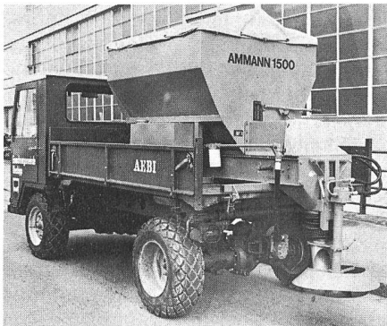
Aufsetzstreuer Ammann 1500 für Kommunalfahrzeuge, Behälterinhalt 1,5 m 3
