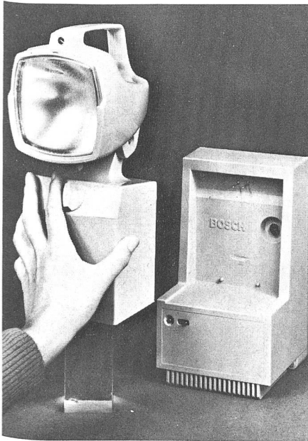
Ein Bosch-Handscheinwerfer, kombiniert mit einem Ladegerät und eingebautem Netzwärter, stellt eine sichere Notbeleuchtung dar
