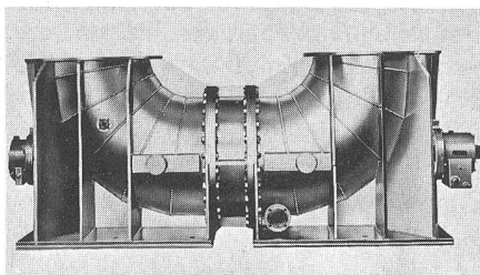
▲ Umwälzpropellerpumpe Baugrösse 900 mm
