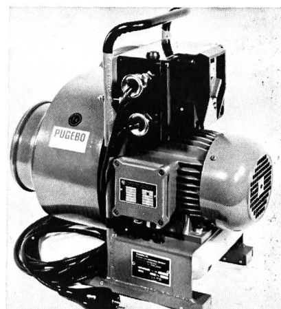
Ex-geschützt SEV-geprüft. Leistung 40 oder 60 m 3 , 220 Volt
