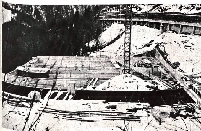
Abb. 2. Blick talauswärts. Im Bild rechts oben Strasse nach Engelberg und darüber das Trasse der Luzern-Stans-Engelberg-Bahn. Im Vordergrund die alte mechanische Kläranlage. Bauzustand Ende 1974
