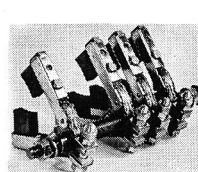
Schleifringkörper und Bürstenhalterelemente auch als Sonderausführungen
