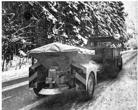
Salz- und Splittstreuer-Anhänger AMA-6H und 15H Inhalt 750 l und 1500 l
