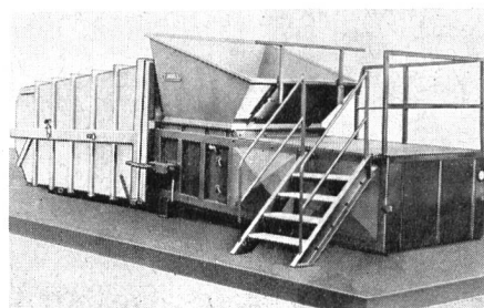
Kehrichtpresse Turner
