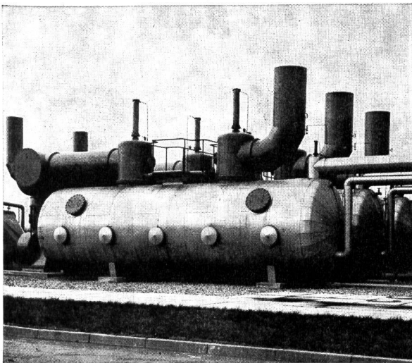
Rückgewinnung von Kohlenwasserstoffen in Klebeband-Produktion
