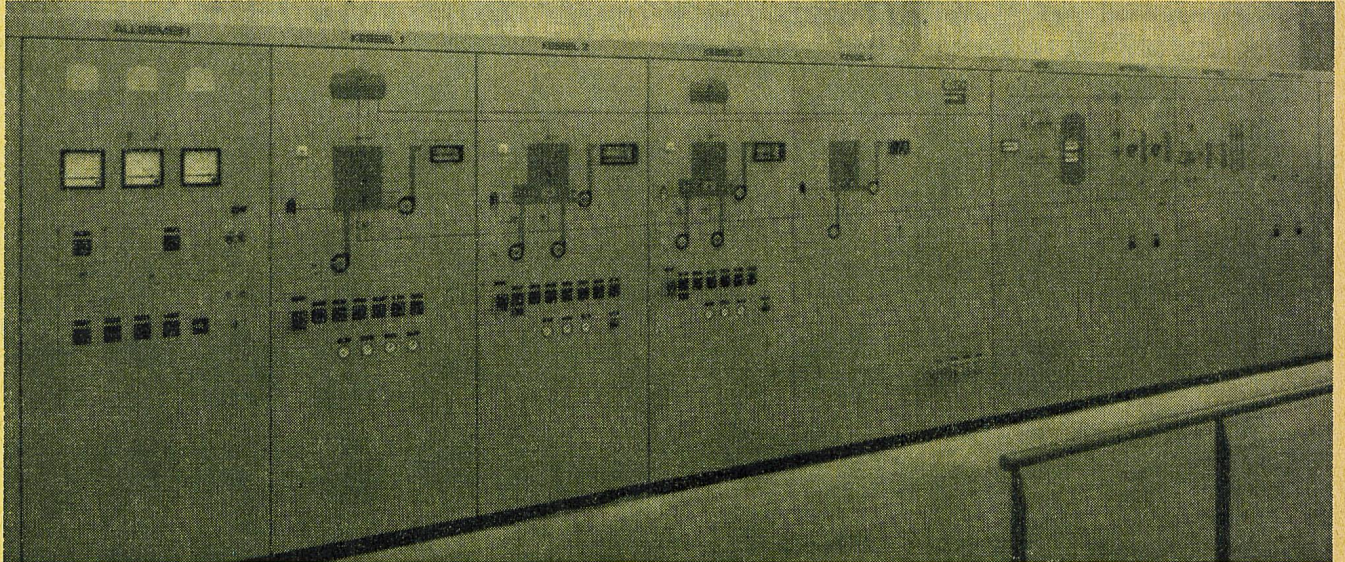
Steuer- und Alarmtableau für die Elco-Feuerungsanlage im Versandhaus Jelmoli, Otelfingen
