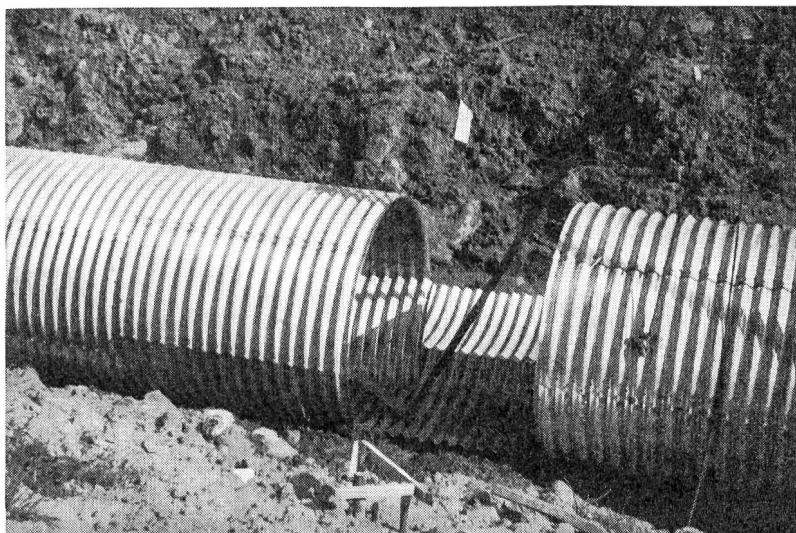
Krebsbacheindolung im Kanton Thurgau, Kreisprofil \varnothing 1,83 m, 161 m lang
