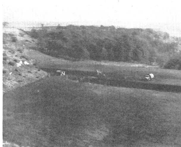
Abb. 1. «Controlled Tipping» in Bradford, England. (Bild durch Vermittlung von Mr. U. Parrat, Director of Public Cleaning.)
