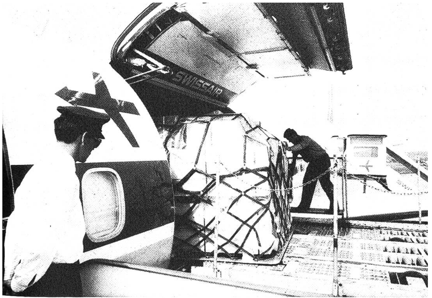
Paletteneinlad – ein kombiniertes Passagier/Frachtflugzeug DC-8-62F transportiert 80 Passagiere und 7 Paletten.
