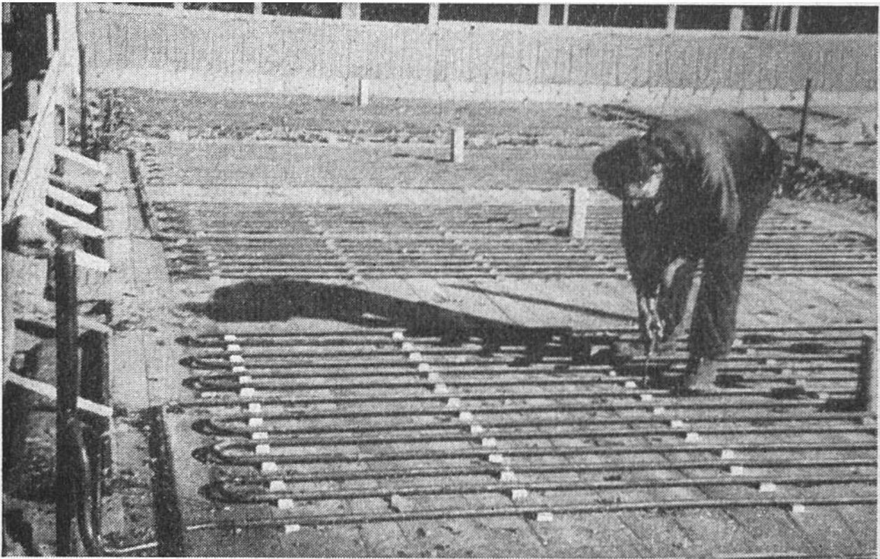
Montage einer Strahlungsheizung (System Crittall). Die Röhren, durch die später warmes Wasser fließt, werden in der Decke verlegt. Darüber kommt eine Eisenbetonschicht mit Abdichtung gegen den Fussboden des folgenden Stockwerkes.
