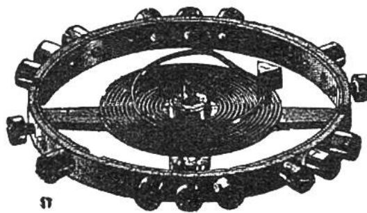
Unruhe mit eingesehter Spiralfeder einer Taschenuhr Zenith
