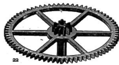
Zwischenrad mit Trieb
