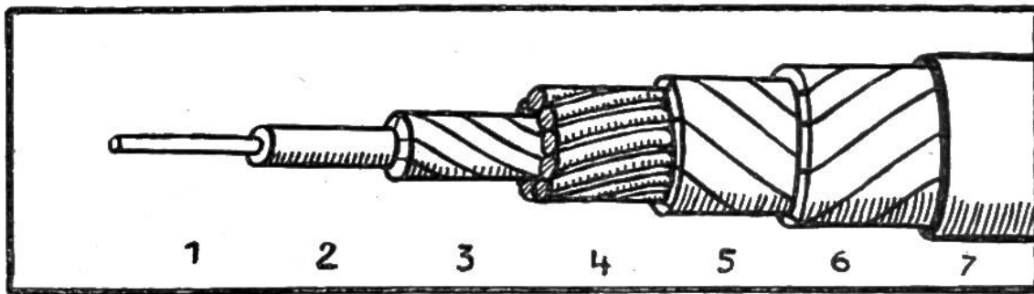
Die Bestandteile eines Unterseekabels. 1. Leitung aus Kupfer. 2. Guttapercha-Isolation. 3. Jute. 4. Eiserner Schutz- und Tragdrähte. 5. Jute. 6. Jute. 7. Geklebte Schutzschicht.
