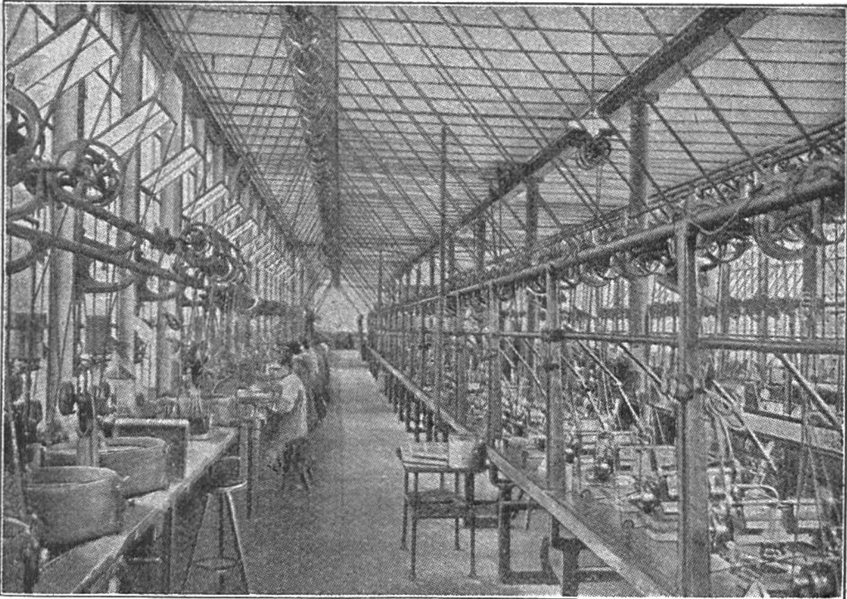
Teilanblick eines Arbeitsraumes „Zenith“ für Stahlstücke.
