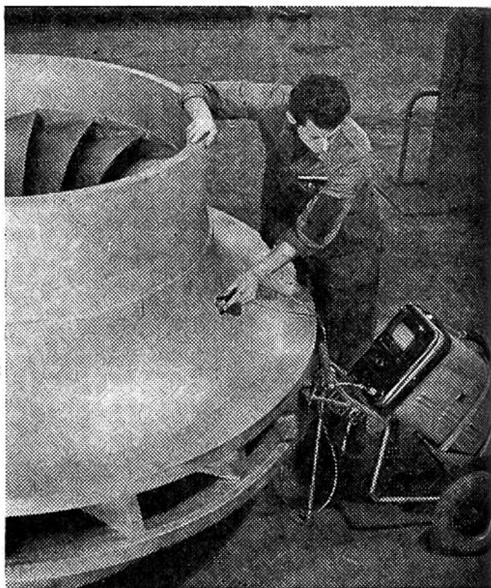
Ein Laufrad einer Francis-Turbine wird mit Ultraschall geprüft.
