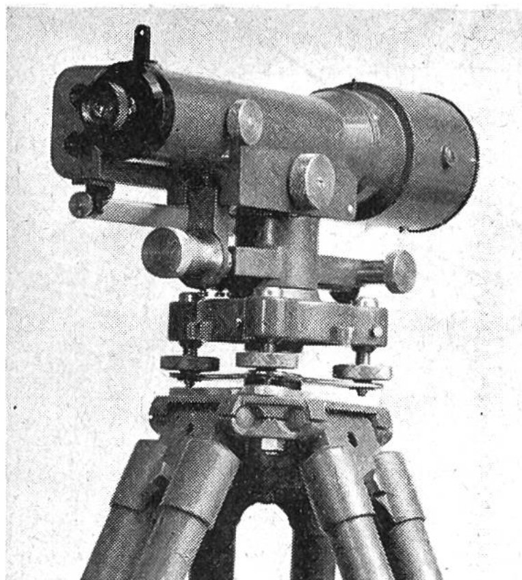
Nivellierinstrument.
