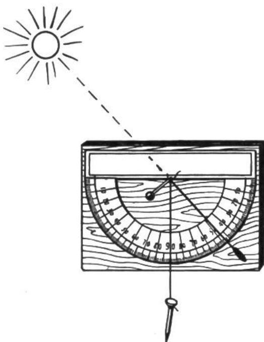
Selbstgebastelter Winkelmesser
