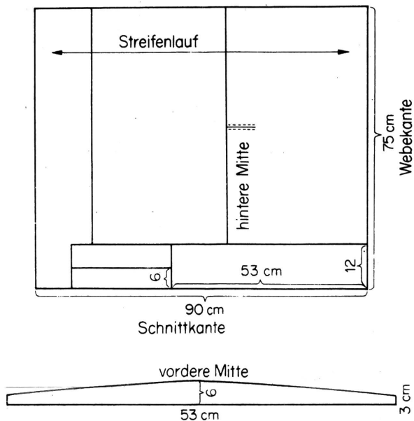
Oberteil des Kinder - Kleidchens Abänderung
