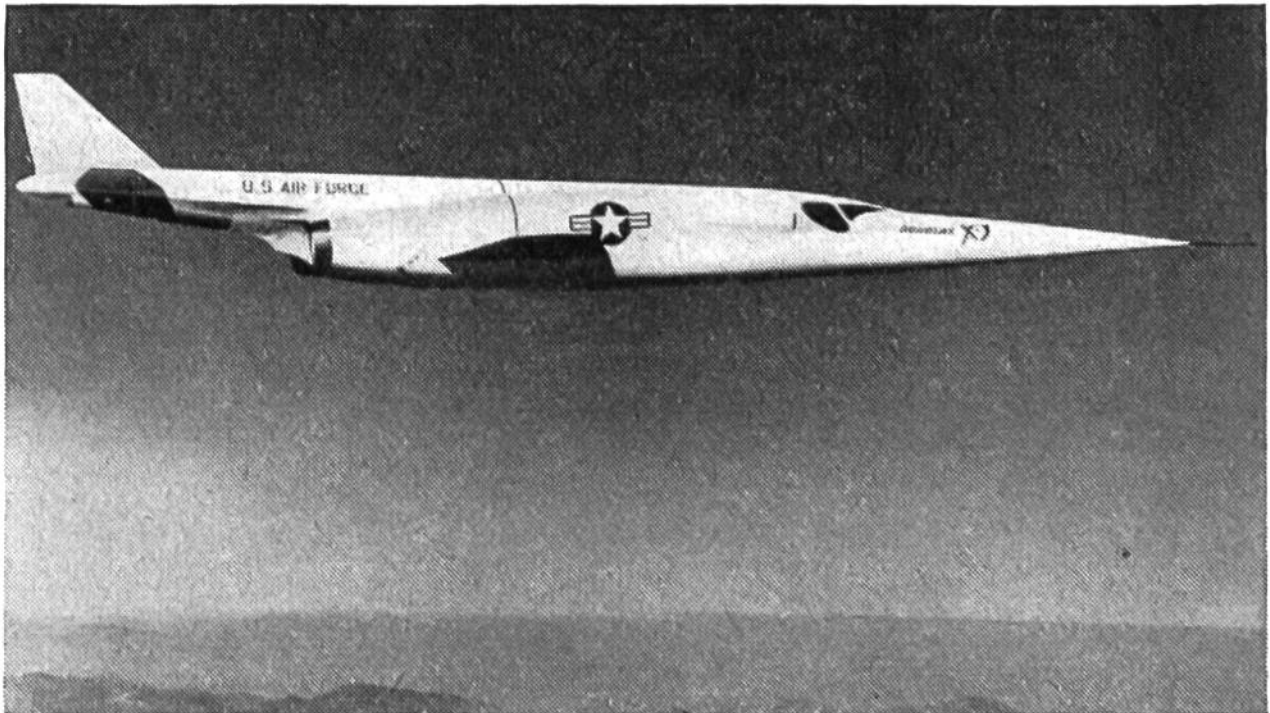
1956: Forschungsflugzeug Douglas X-3, errechnet für 3fache Schallgeschwindigkeit, entsprechend ca. 3200 km/h in sehr grosser Höhe. Spannweite 6,9 m. Fluggewicht über 12000 kg. 2 Düsentriebwerke von 4080 kg Schub, in späterer Erprobungsphase 8000 kg entsprechend ca. 36000 PS bei 1200 km/h.
