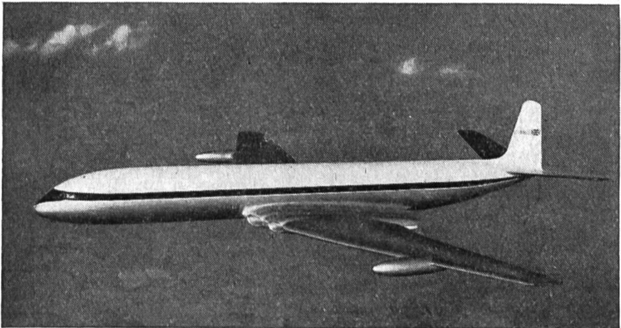
1956: Comet IV, 4motoriges Düsenverkehrsflugzeug für 60–76 Passagiere in Druckkabine. Spannweite 35 m, Fluggewicht 70000 kg. Reisegeschwindigkeit 800 km/h. Motorleistung 18144 kg Schub, entsprechend ca. 53000 PS bei 800 km/h. Reichweite 4800 km.
