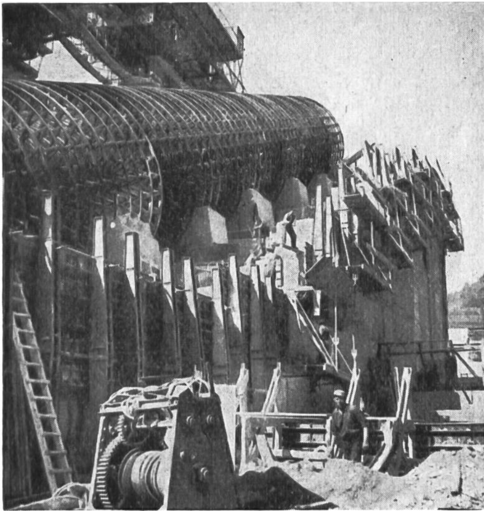
So wurden die beinahe sechs Meter weiten Druckleitungen in die Stau- mauer einbetoniert. Die Rippen dienten zur Versteifung der Rohre, die sonst durch das Gewicht des Betons zusammengepresst worden wären.
