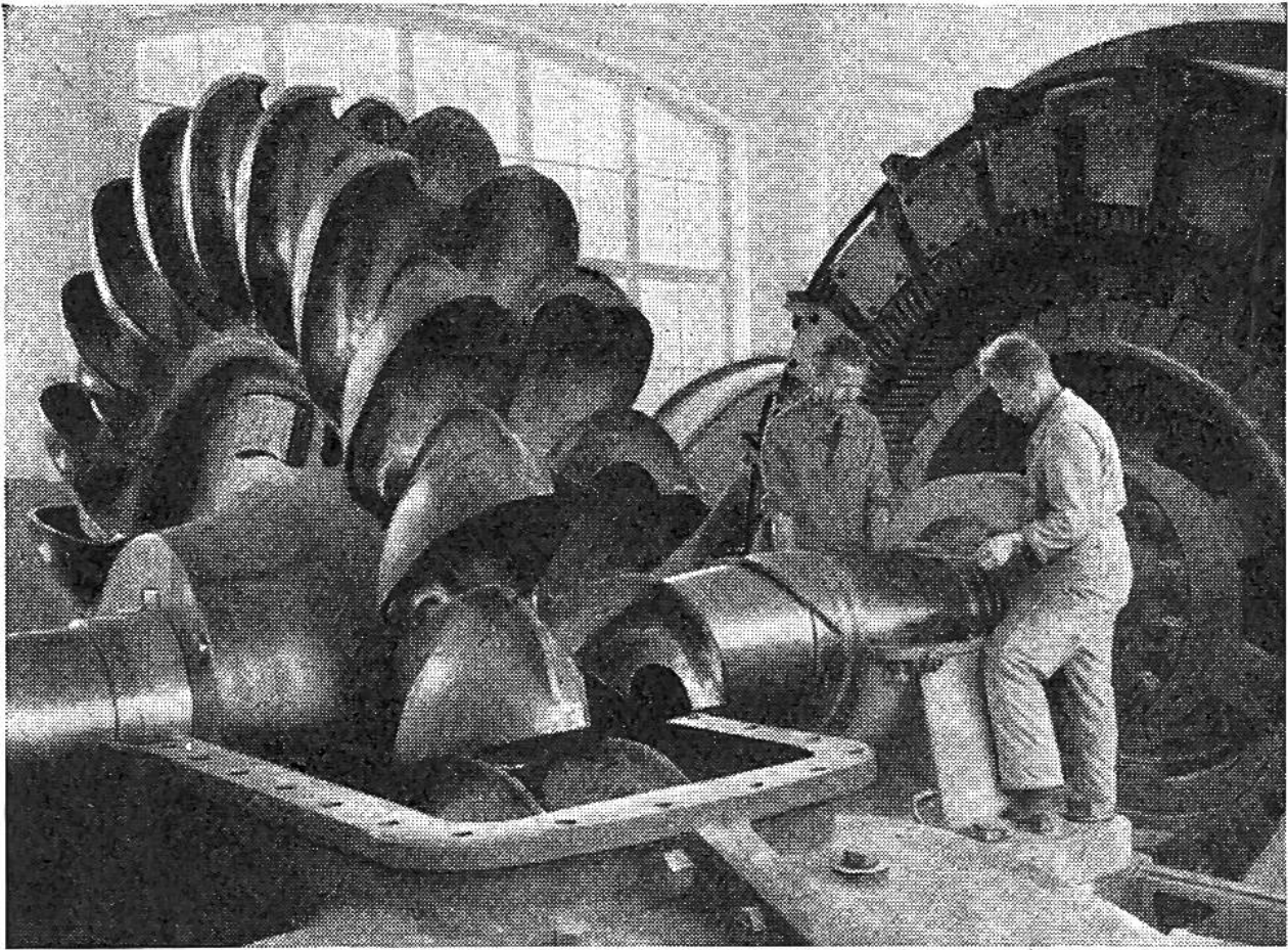
Eine der zwei Pelton-Turbinen mit den mächtigen Schaufeln und der dazu gehörige Generator (Stromerzeuger) im Hochdruck-Speicherkraftwerk Lucendro während des Baus. - Vom Stausee her stürzt das Wasser in einer Druckleitung auf die 930 m tiefer gelegenen Turbinen-Schaukeln der Zentrale Airolo. Diese Turbine schluckt 3 Kubikmeter Wasser in der Sekunde und leistet 33 000 PS.
