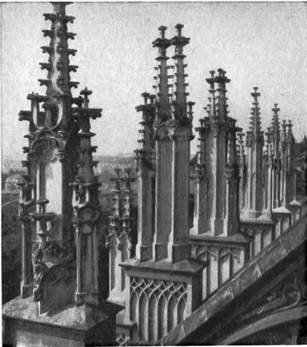
Die ersetzten Strebeböcker mit ihren Turmaufbauten am Berner Münster.
