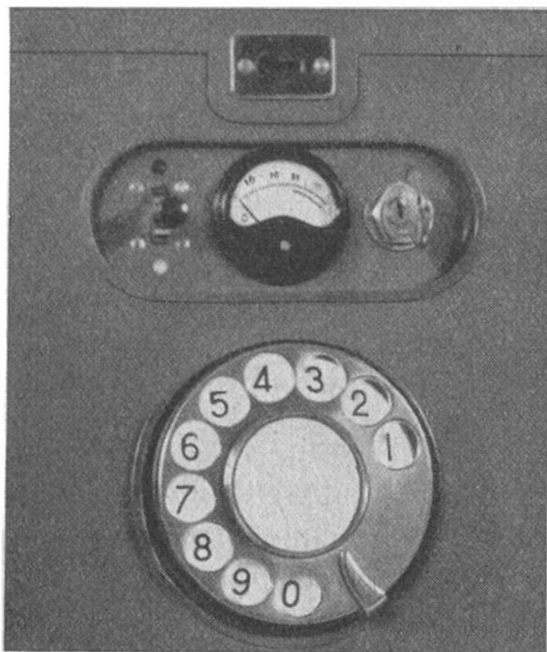
Teil eines Telephon-Apparates für drahtlose Telephonie. Oben: Schalter und Messinstrument zur Kontrolle der Batterien, Schloss zum Abschiessen gegen unbefugte Benützung des Apparates. Unten: Wählscheibe.
