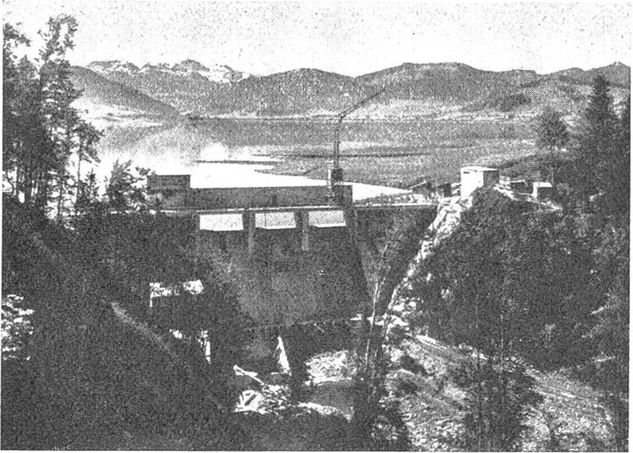
Die Staumauer „in den Schlagen“ bei Einsiedeln. Schon stauen sich die Wasser zum zukünftigen See. Die Staumauer ist nahezu beendet und lässt die drei Öffnungen des Überfallwehres für das überflüssige Wasser erkennen.
