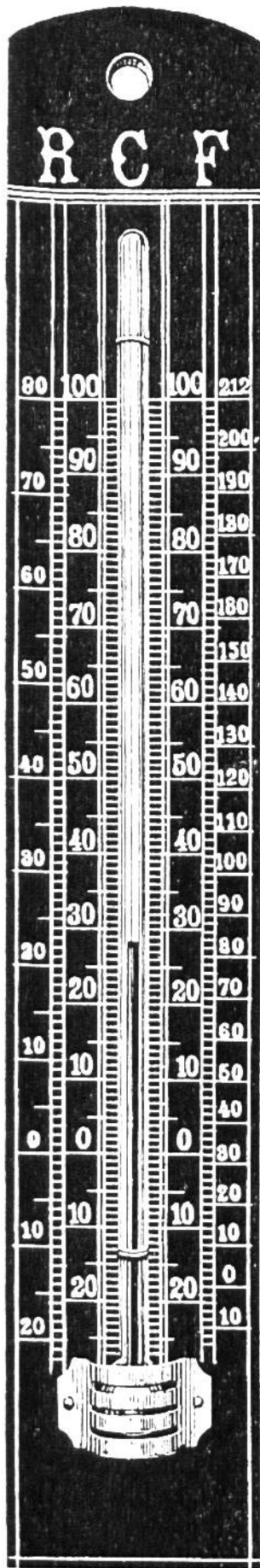
Réaumur-Celsius-Fahrenheit
