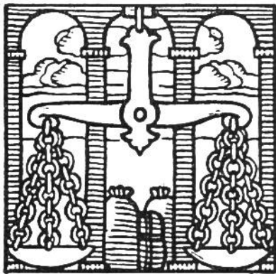
Sternbild Waage
