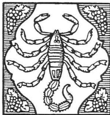
Sternbild Skorpion
