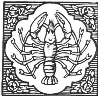
Sternbild Krebs
