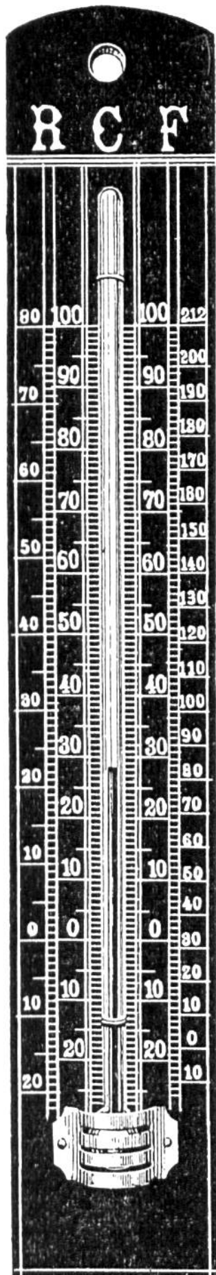
Réaumur-Celsius-Fahrenheit
