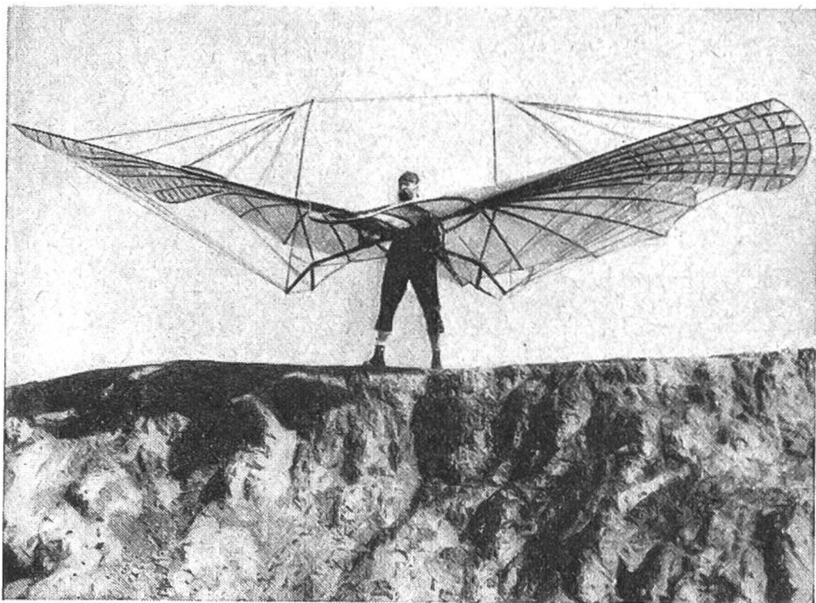
Lilienthals letztes Flugzeug, welches er noch kurz vor seinem Tode herstellte. Es war ein vergrößerter Gindeder mit Schlagflügelwerk, das durch einen Kohlen säuremotor, den er auf dem Rücken trug, getrieben wurde.
