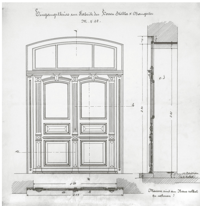
Plan der Eingangstüre zur Fabrik Stettler & Bangerter.
