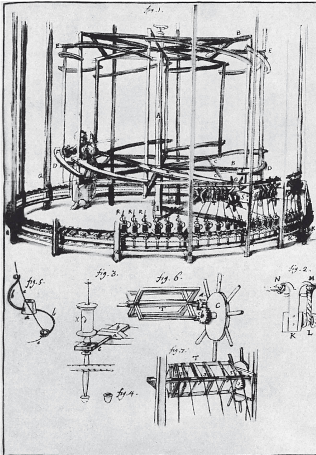
Zwirnrad mit «Radmeitli». Zeichnung von Christoph Martin, 1745
