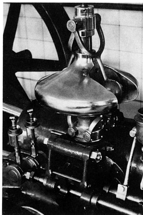
Sulzer-Dampfmaschine mit Bodmer-Steuerung (Detail)
