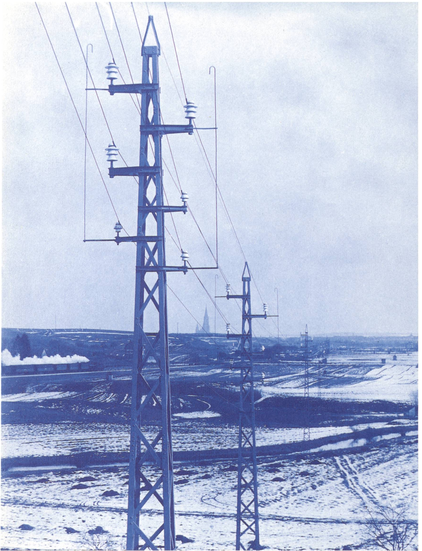
Gittermastenleitung Ulm-Trochtelfingen 1915 durch Kummeler & Matter, Stuttgart, für den Bezirksverband Oberschwäbischer Elektrizitätswerke Biberach (O.E.W.) erstellt: Masten mit Fangbügel für Leitungs- und Bahnkreuzungen. Im Hintergrund fährt ein Dampfzug nach Ulm, dessen Münster zu erkennen ist (Original-Blaukopie, Dokument Nr. 1979).
