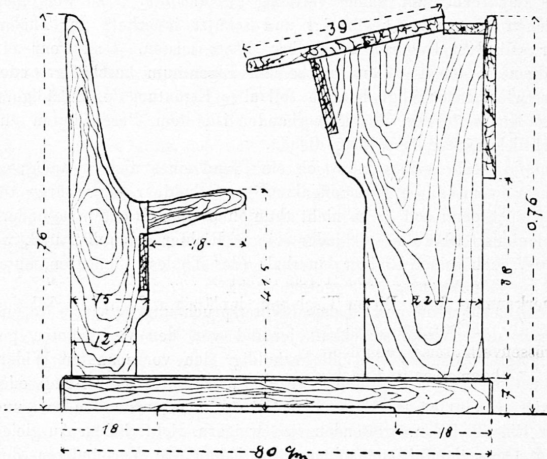
Maassstab 1:10.
