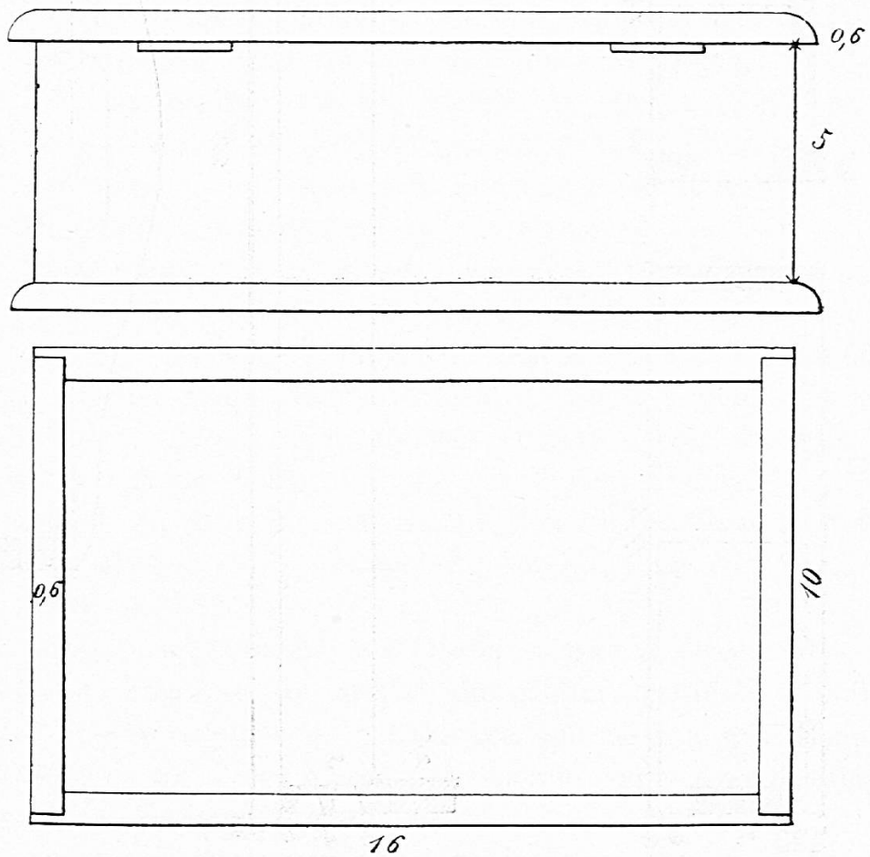
Fig. 37. Kassette, überpl.
