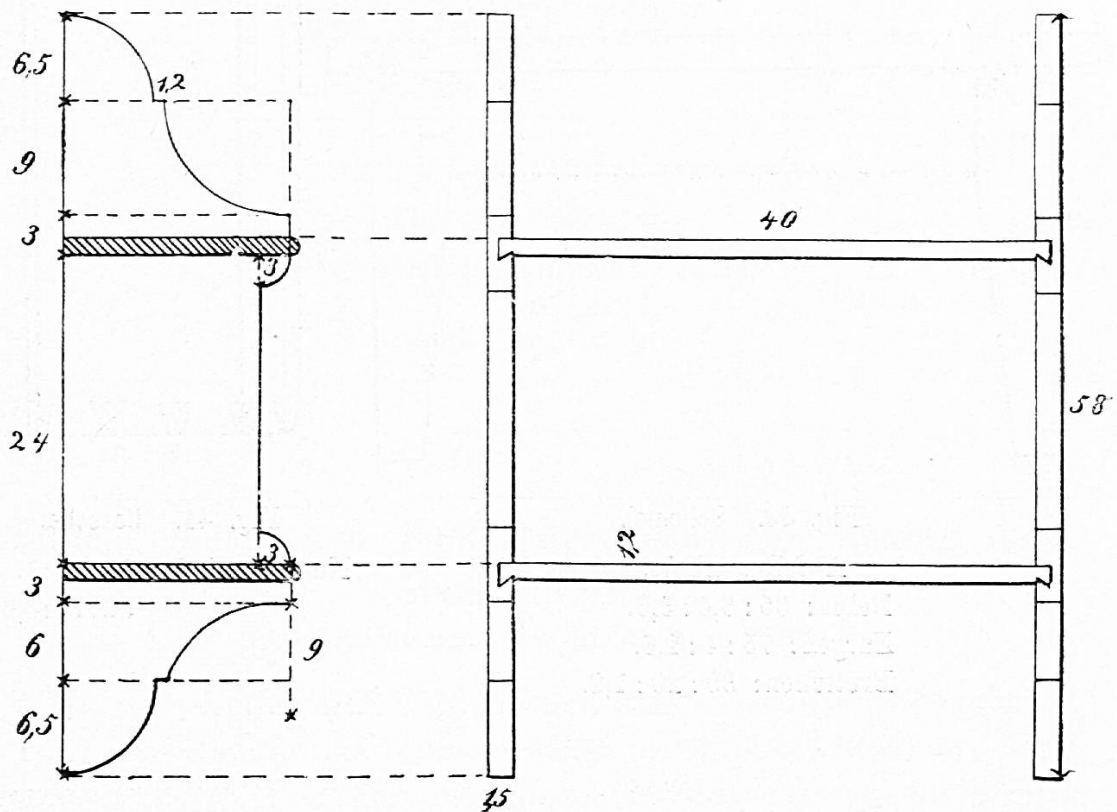
Fig. 39. Bücheretagère. Tannenholz: 120 : 17 : 1,8. 90 : 18 : 1,5.
