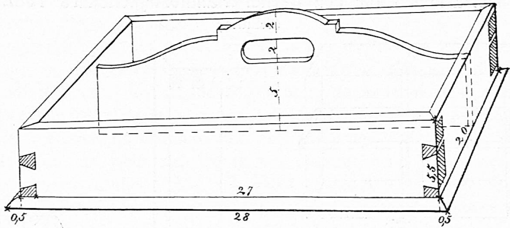
Fig. 36. Servicekasten.
