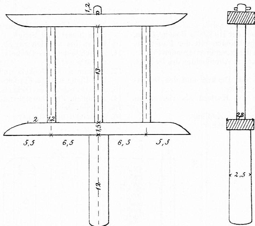
Fig. 25: Schnurhaspel. Buchenholz: 30 : 10 : 3. (Fortsetzung folgt.)
