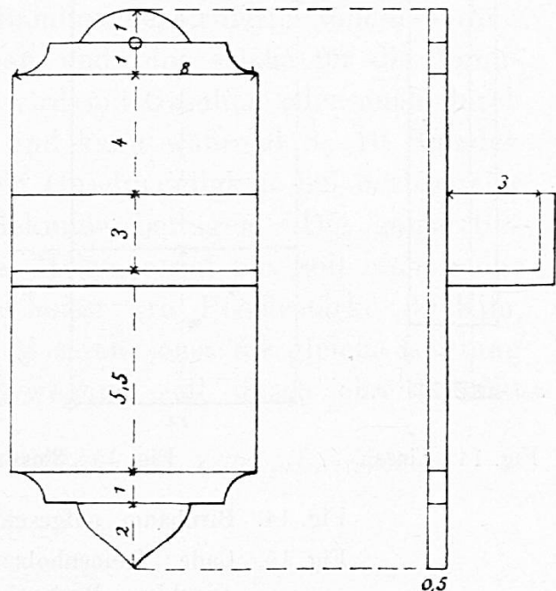
Fig. 19. Zündholzbehälter.
