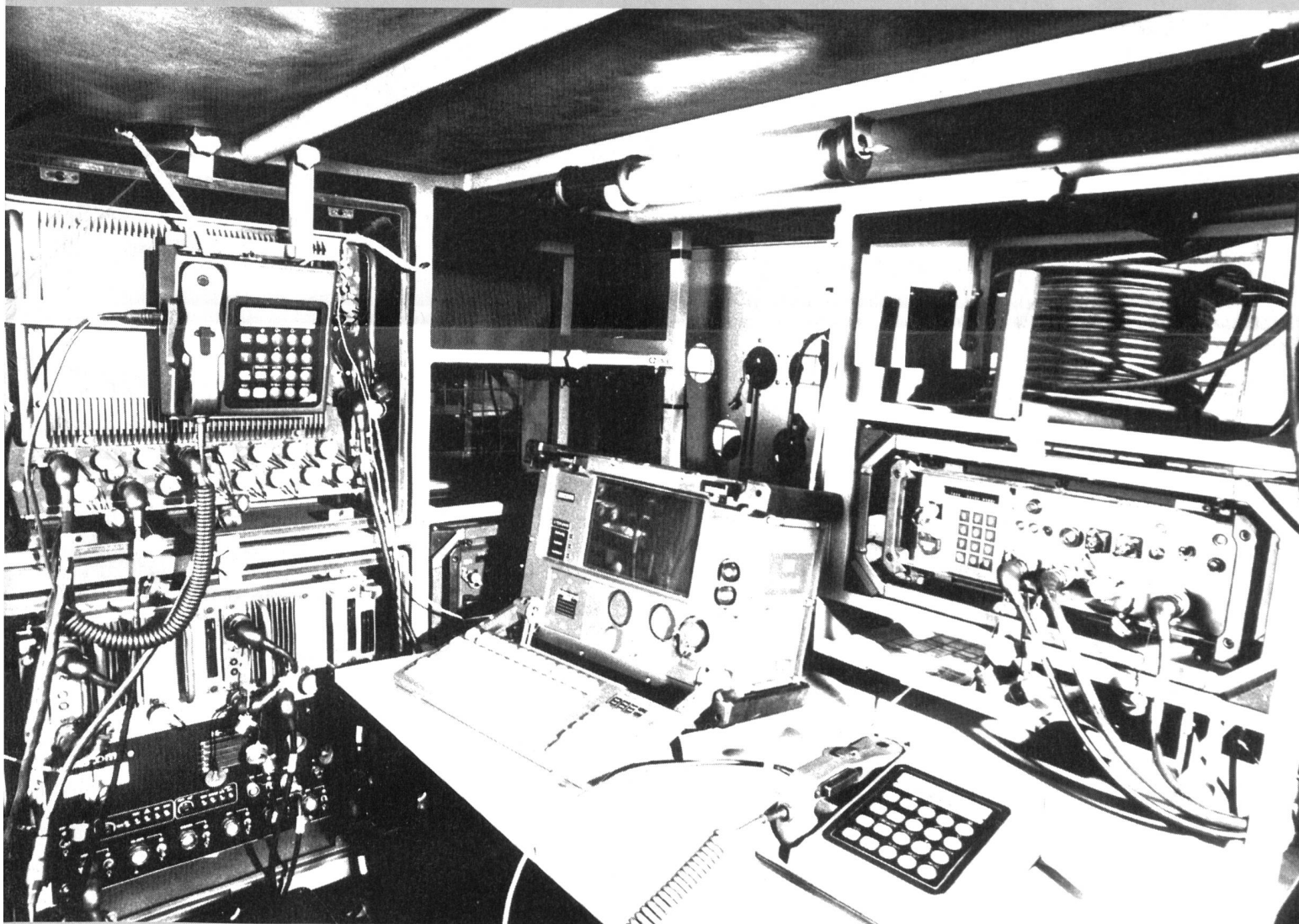
Das innere eines IMFS- Vermittler-Fahrzeugs
